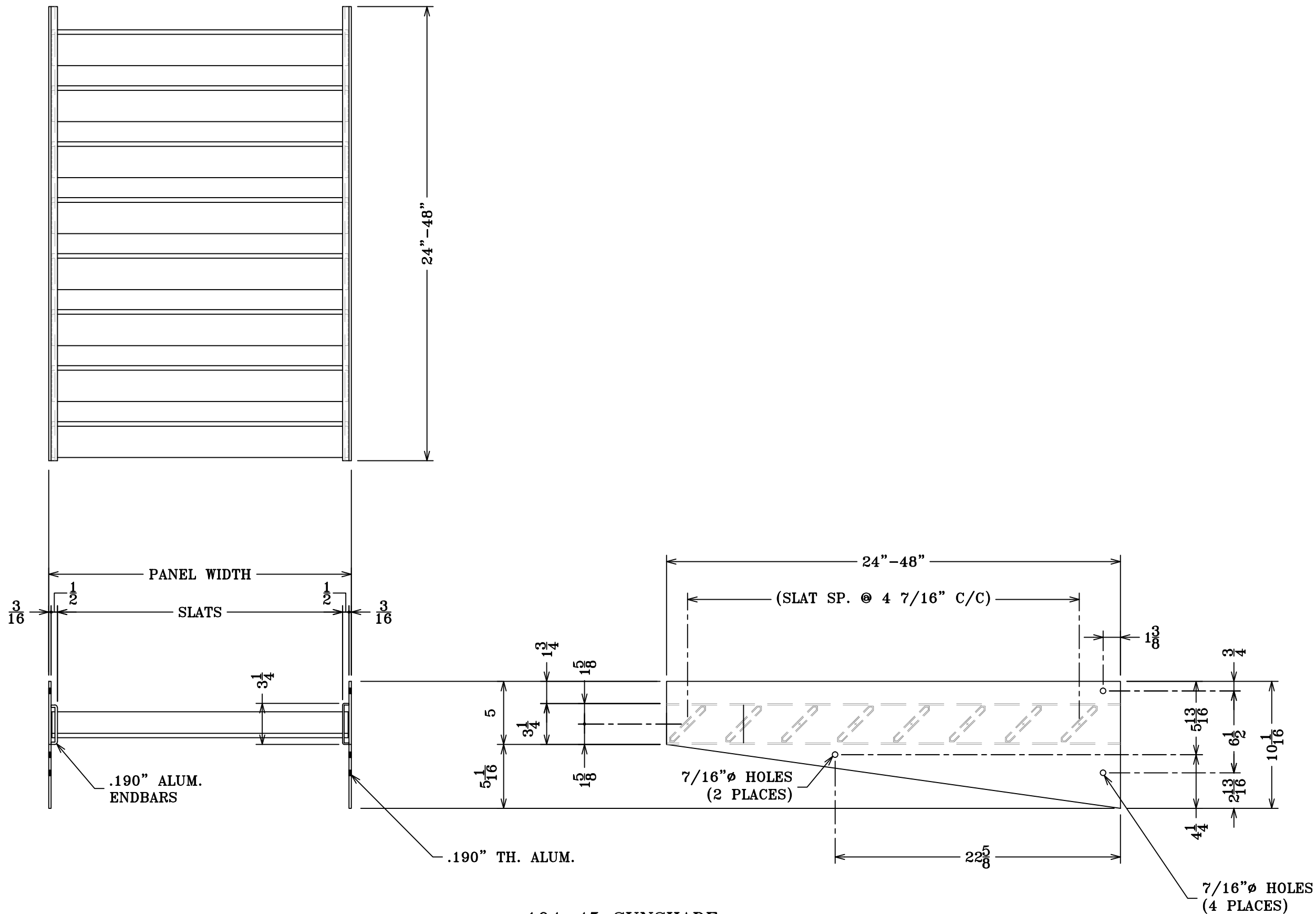
104-45 SUNSHADE
